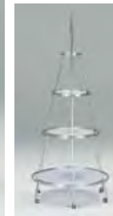
■円錐タワーアクリル棚型 本体：W750×D750×H1800 (58105) 丸棚：大 Ø750 中 Ø550 小 Ø350 (58106) 仕様：ステンレスフレーム 丸棚 / ステンレス枠アクリル板 ステンレスポトルフック (58107)
