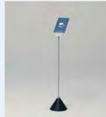
■メッセージスタンド W210×D210×H890 (63210) 仕様：スチールパイプ / クロームメッキ
